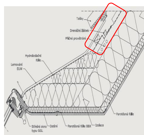
Obr. 2) průřez kontralaty, zdroj www.velux.cz
