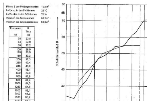
Obr. 8) ukázka naměřených hodnot vzduchové neprůzvučnosti, zdroj Pavatex SA
