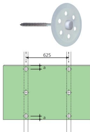
Obr. 12: Ejothem STR H se zátkou a schéma kotvení desek Pavatex (rozměr)
