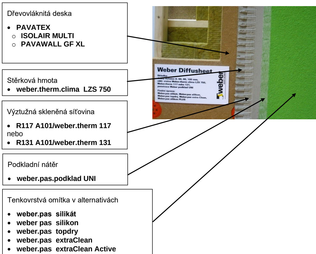
Obr. 13: Omítkové souvrství WEBER zateplovacího systému WEBER – diffusheet®
